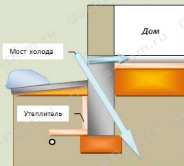
Мостик холода через неутепленную надземную часть фундамента и отсутствие боковой теплоизоляции плавающего пола
