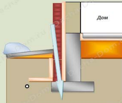
Мостик холода через кирпичный фасад
