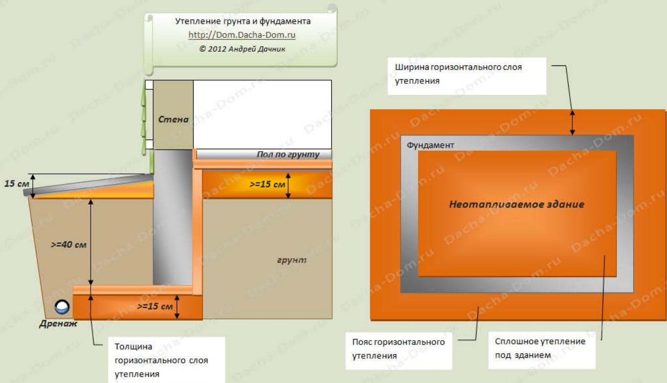
Схема № 38 Схема утепления неотапливаемого в холодный период здания на пучинистых грунтах*
