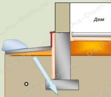
Мостик холода через бетонную подготовку при отсутствии горизонтального утепления
