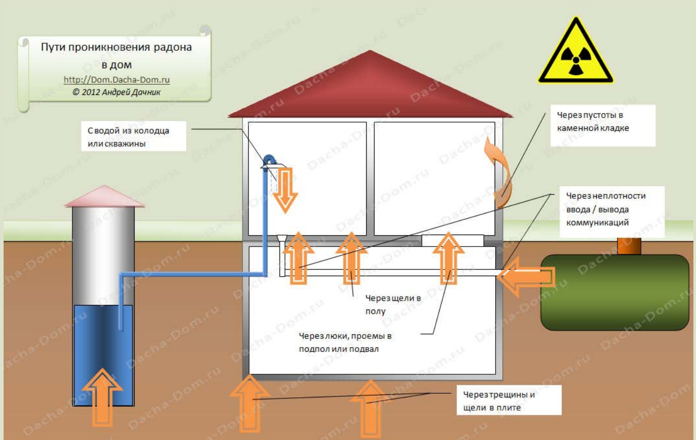
Схема №8. Пути проникновения радона в жилой дом.
