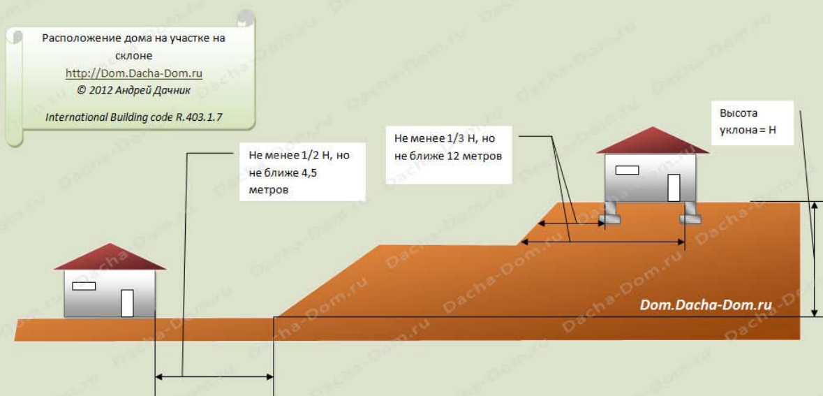
Схема №45. Схема рекомендуемого расположения дома вблизи склона по нормам IBC/IRC-2012.
