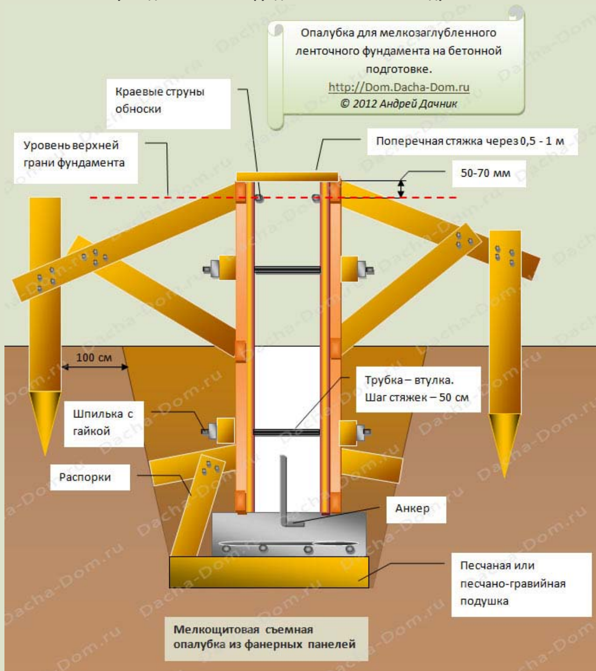
Схема №22. Опалубка для ленточного фундамента на бетонной подушке.
