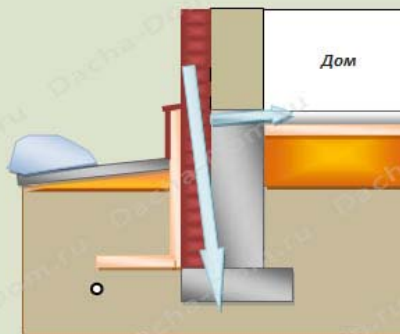
Мостик холода через кирпичный фасад и отсутствие боковой теплоизоляции плавающего пола
