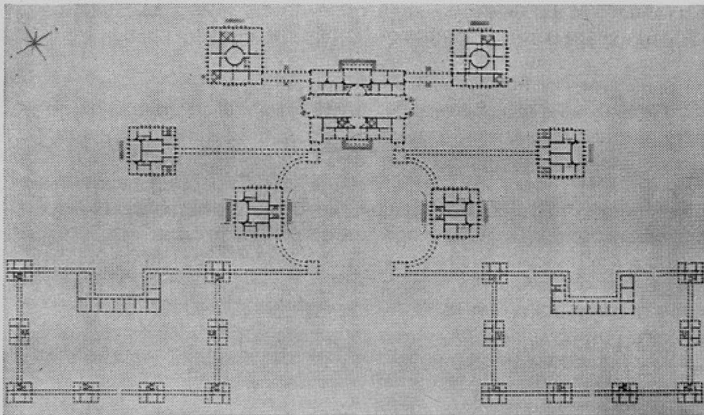
И. Старов. Дворец в Пелле. План (копия). 1784—1789.
